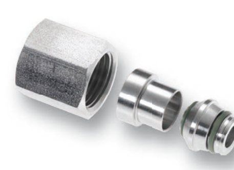
37度扩口接头
